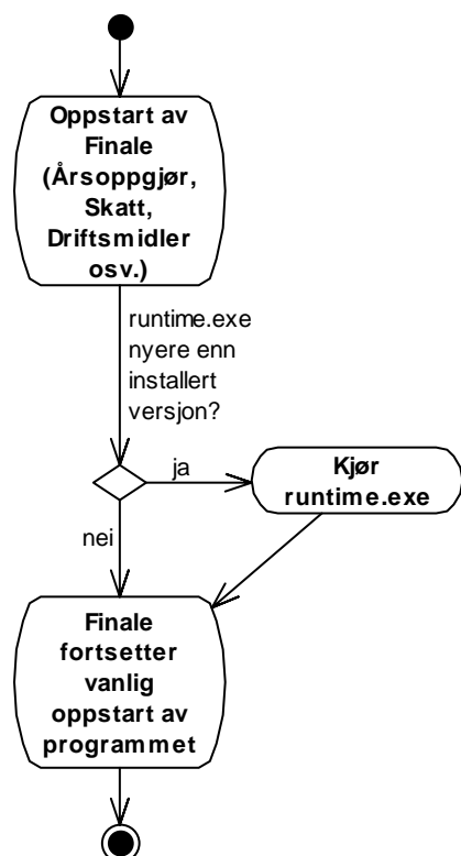
Fig. 2.1 Programmets sjekk av installerte systemkomponenter ( runtime.exe ) ved oppstart.
