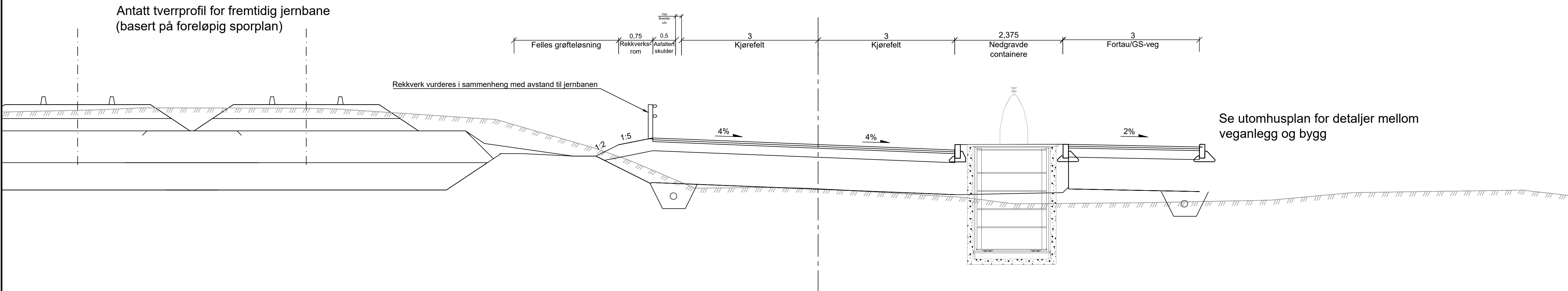
Normalprofil Havnevegen Med nedgravde containere
