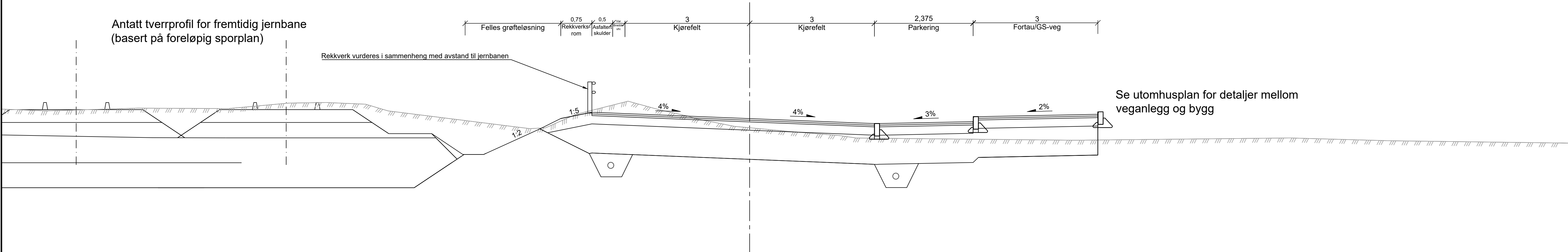
Normalprofil Havnevegen Med langsgående parkering
